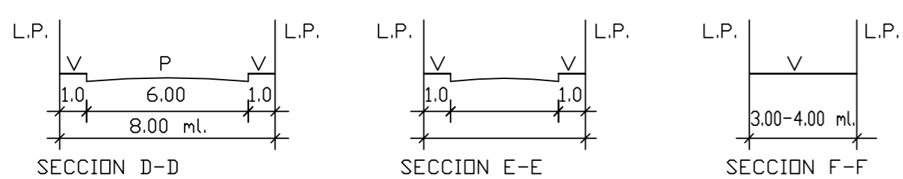
SECCION D-D
