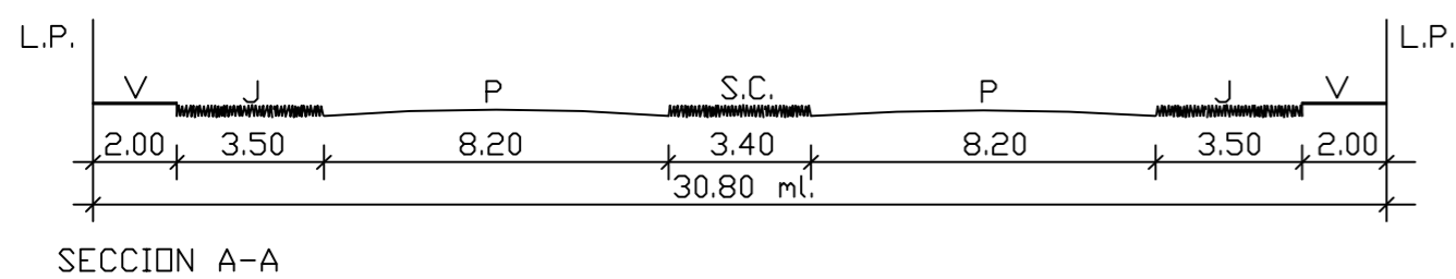
SECCION A-A
