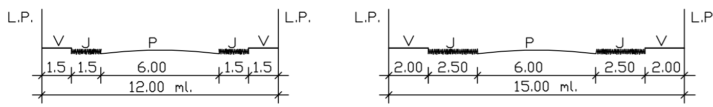
SECCION B-B
